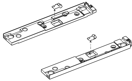
1. Atskirkite kairįjį ir dešinįjį tvirtinimo elementus nuo atitinkamų laikiklių.
