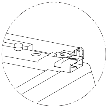
2. Padėkite kairįjį ir dešinįjį laikiklius ant skalbyklės viršutinio dangčio. Pagal kairėje esantį papildintą vaizdą, tiksliai įstatykite kairįjį ir dešinįjį laikiklius ties skalbyklės priekine ir šonine pakopa. Priveržkite kairįjį ir dešinįjį laikiklius 3 varžtais per vidines tvirtinimo angas, kaip parodyta papildintame vaizde dešinėje.
