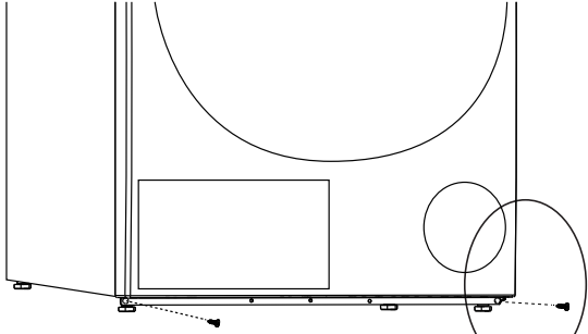
3. Išsukite 2 varžtus džiovyklės priekinio skydelio apačioje.
