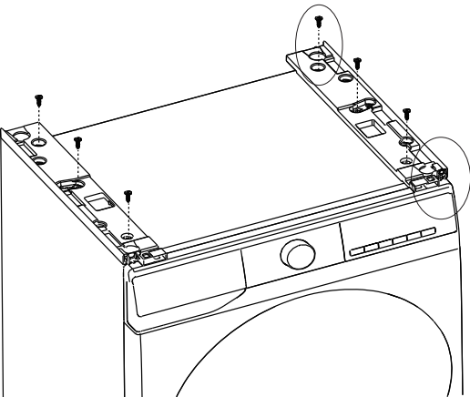
2. Padėkite kairįjį ir dešinįjį laikiklius ant skalbyklės viršutinio dangčio. Pagal kairėje esantį papildintą vaizdą, tiksliai įstatykite kairįjį ir dešinįjį laikiklius ties skalbyklės priekine ir šonine pakopa. Priveržkite kairįjį ir dešinįjį laikiklius 3 varžtais per vidines tvirtinimo angas, kaip parodyta papildintame vaizde dešinėje.
