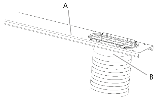
A. Išorinė slankiklio dalis B. Lango adapteris
