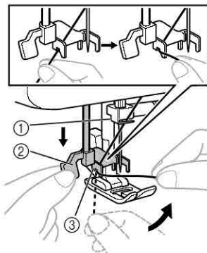
① Иголдержатель ② Рычажок нитевдевателя ③ Направляющая
